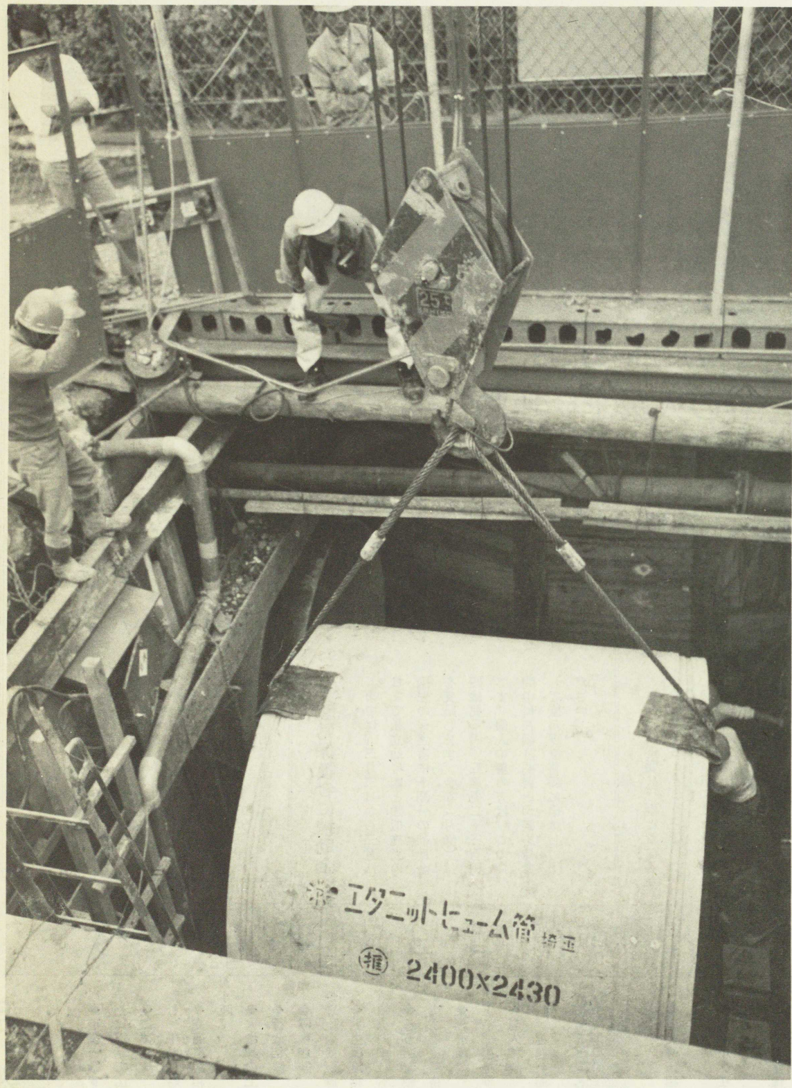
着々と進む下水道工事、クリーン狛江の実現に積極的な水洗化が望まれる
